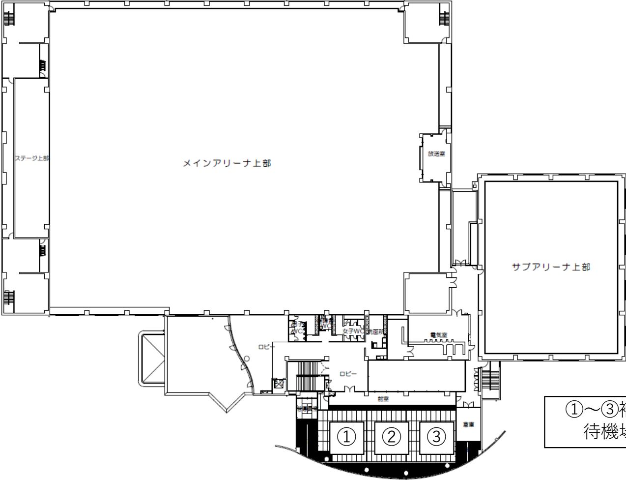
3階平面図 S=1/500
